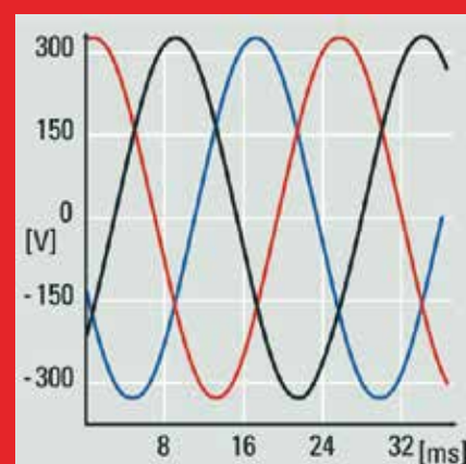
Rara vez se encuentra en la actualidad la situación ideal de la tensión de red senoidal en nuestras redes.
