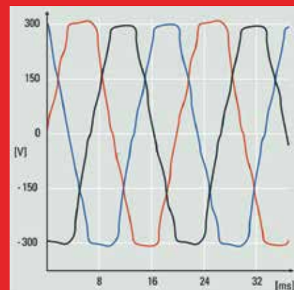
Los cálculos muestran una clara distorsión de la forma de onda de la tensión de red debido a la interferencia de cargas no lineales.
